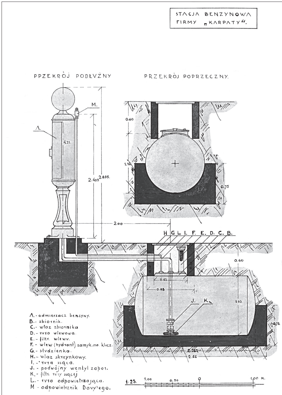
Fotografia 8. Przekrój stacji „Karpaty”
